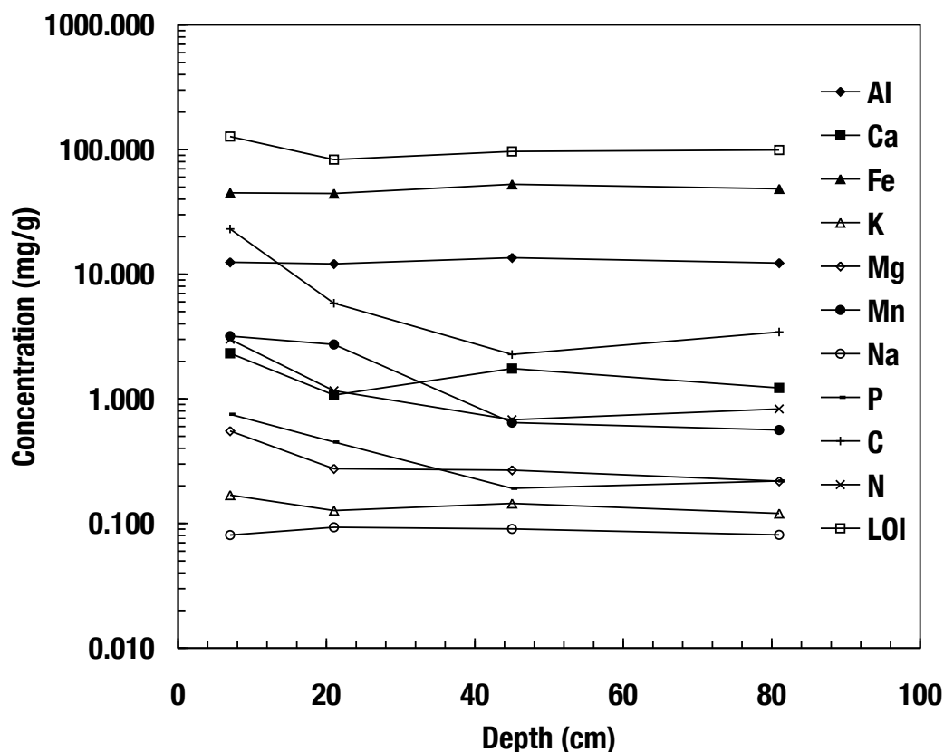
FIGURA 2. Variación con la profundidad en la concentración total de elementos químicos en una calicata excavada en un bosque de Castilla elastica en El Tallonal, Arecibo, Puerto Rico. La escala para los valores de concentración es logarítmica. Los puntos se ubican en el centro de cada uno de los cuatro horizontes observados en la calicata.
