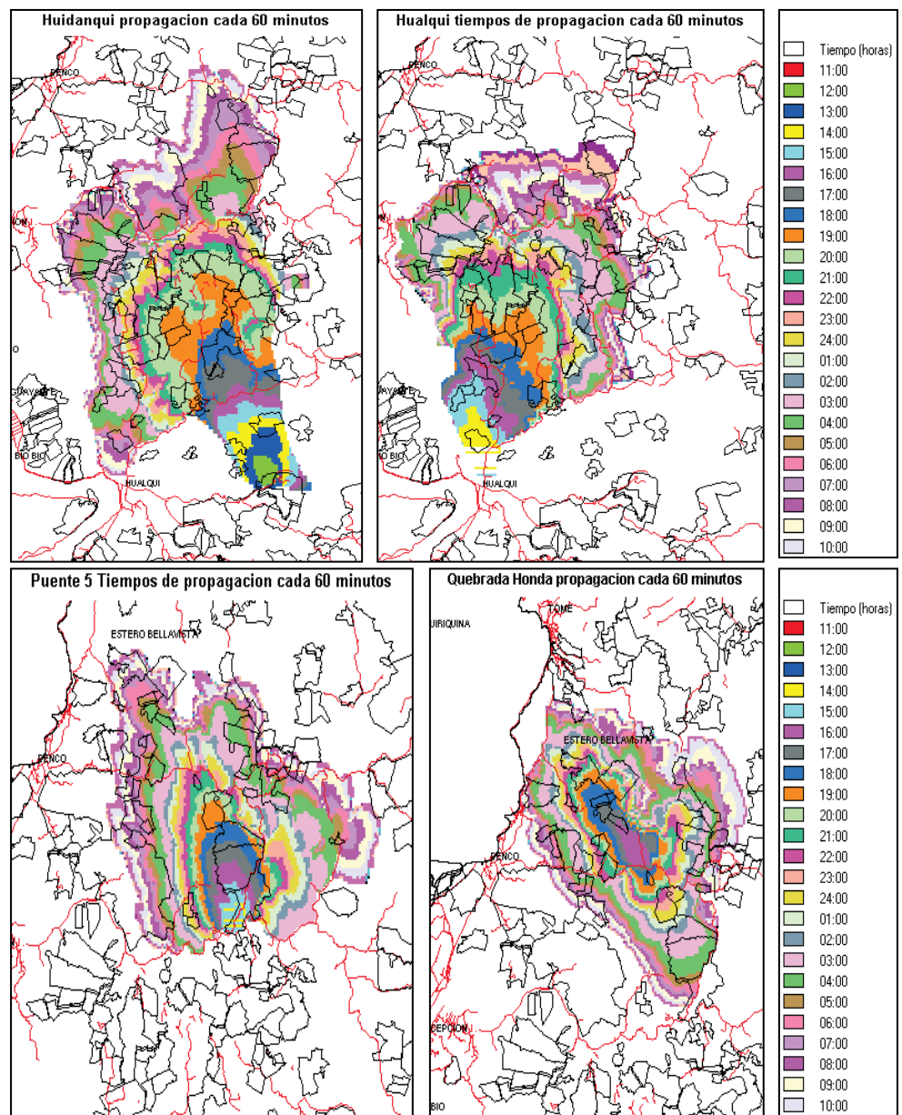
Figura 1 — Simulación de incendios forestales a un período de 24 horas, utilizando el Sistema KITRAL. Las distintas bandas de colores representan cotas de propagación del fuego cada 60 minutos.
